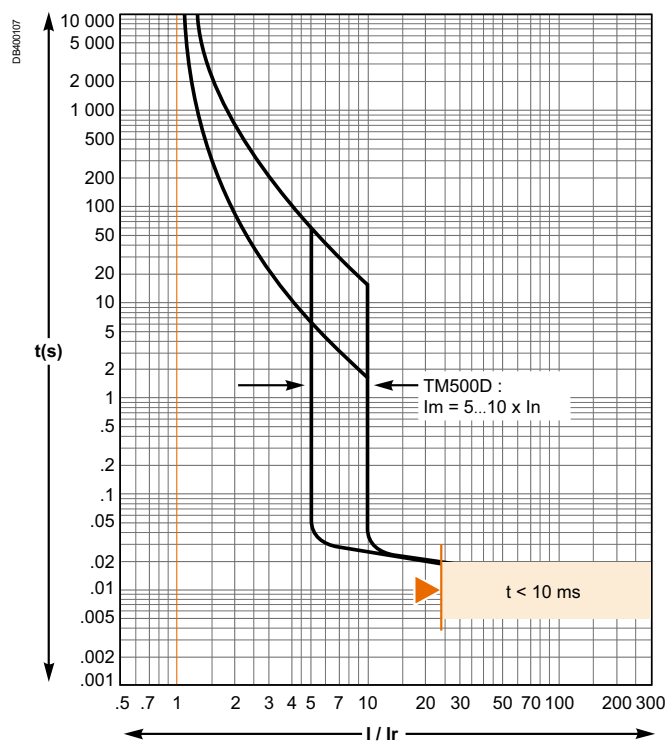
TM500D
