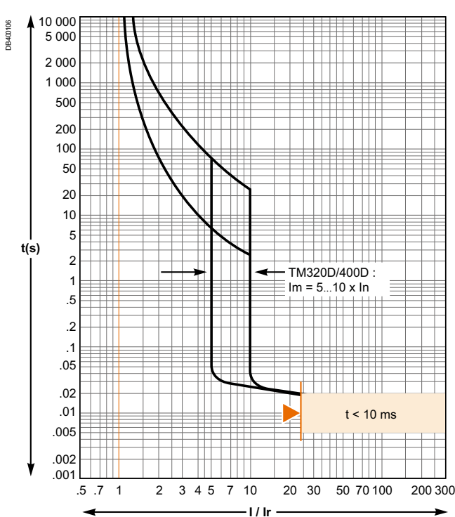
TM320D/400D
