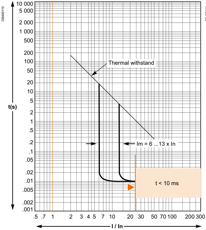
MA320
